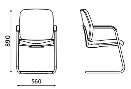
GLOBELINE 5-A
